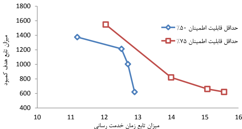
تصویر ۶: تأثیر قابلیت اطمینان بر میزان کمک‌رسانی و زمان خدمت‌رسانی
