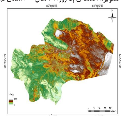
تصویر ۱۳: نقشه‌ی S_1 روز ۱۹۵ سال ۲۰۱۳ استان قم
