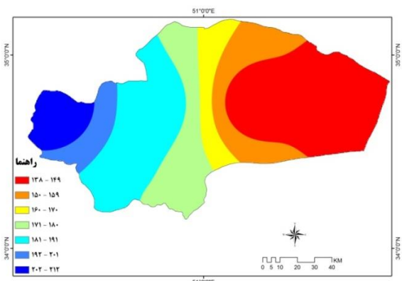
تصویر ۳۳: نقشه‌ی میانگین بارش سالانه‌ی استان قم (۱۹۸۴-۲۰۱۳)
