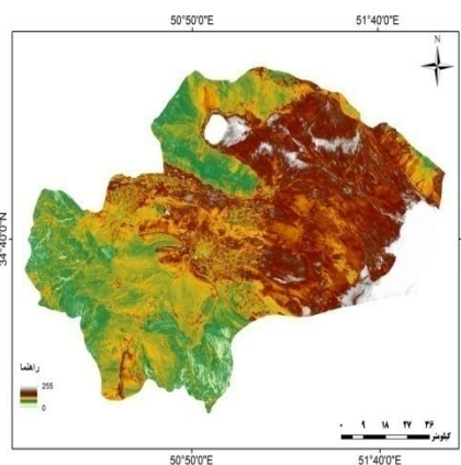
تصویر ۹: نقشه‌ی S_1 روز ۱۸۸ سال ۱۹۸۷ استان قم
