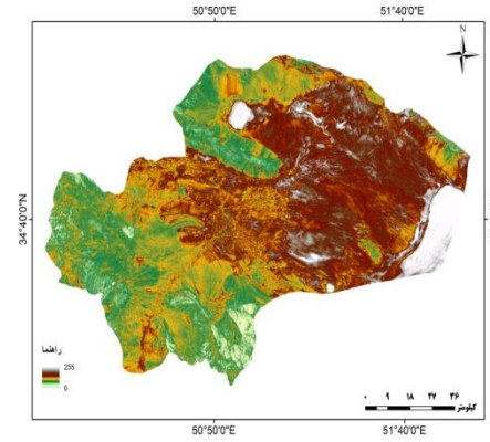
تصویر ۱۷: نقشه‌ی S_2 روز ۱۵۵ سال ۲۰۱۰ استان قم
