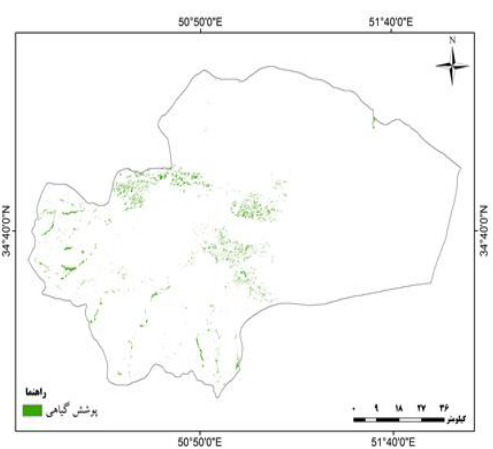
تصویر ۶: نقشه‌ی NDVI روز ۲۰۸ سال ۲۰۰۰ استان قم
