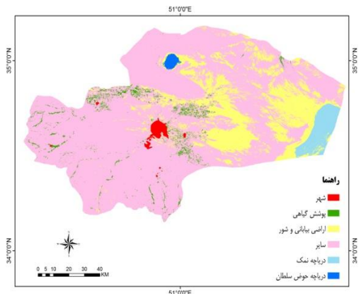
تصویر ۲۵: نقشه‌ی کاربری اراضی سال ۱۹۹۳ استان قم
