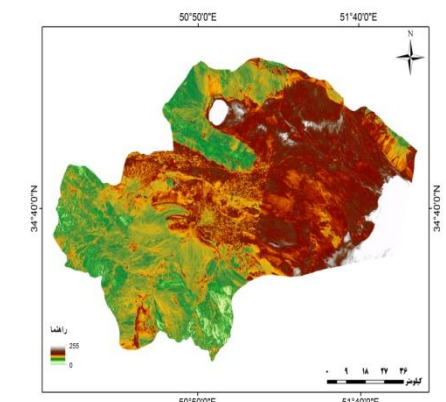
تصویر ۱۴: نقشه‌ی S_1 روز ۱۸۸ سال ۱۹۸۷ استان قم
