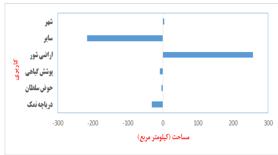
تصویر ۲۹: تغییرات کاربری اراضی استان قم (۱۹۸۷-۱۹۹۳)
