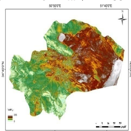
تصویر ۱۱: نقشه‌ی S_1 روز ۲۰۸ سال ۲۰۰۰ استان قم
